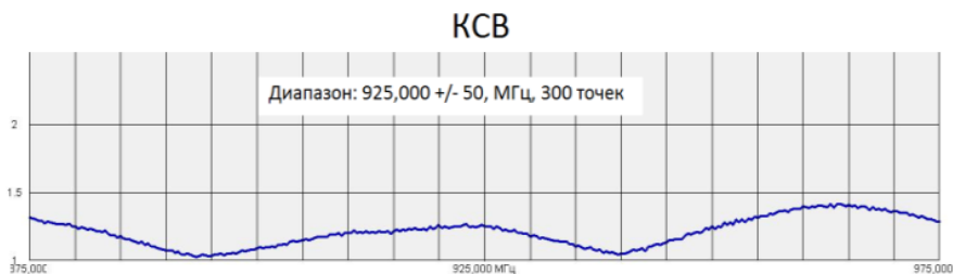
Рисунок 3 - Коэффициент стоячей волны Ксв.
