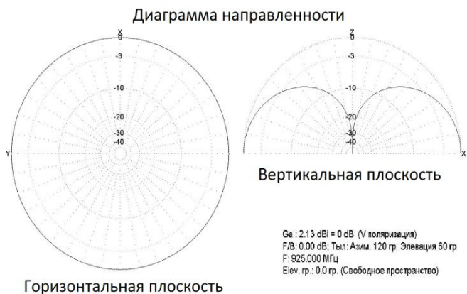
Рисунок 2 – Диаграмма направленности.
